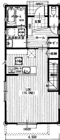
1階 平面図
