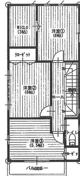
2階平面図
