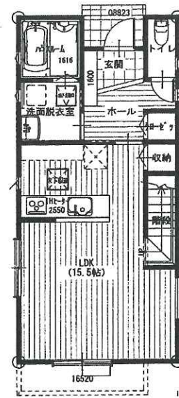
1階平面図
