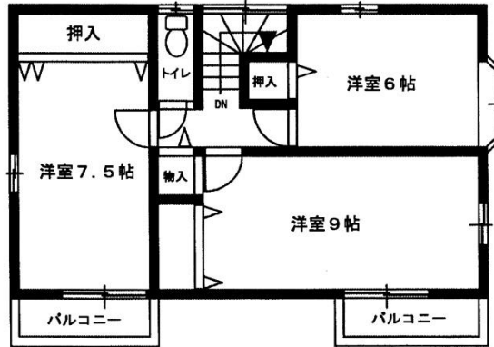
2階間取り図
